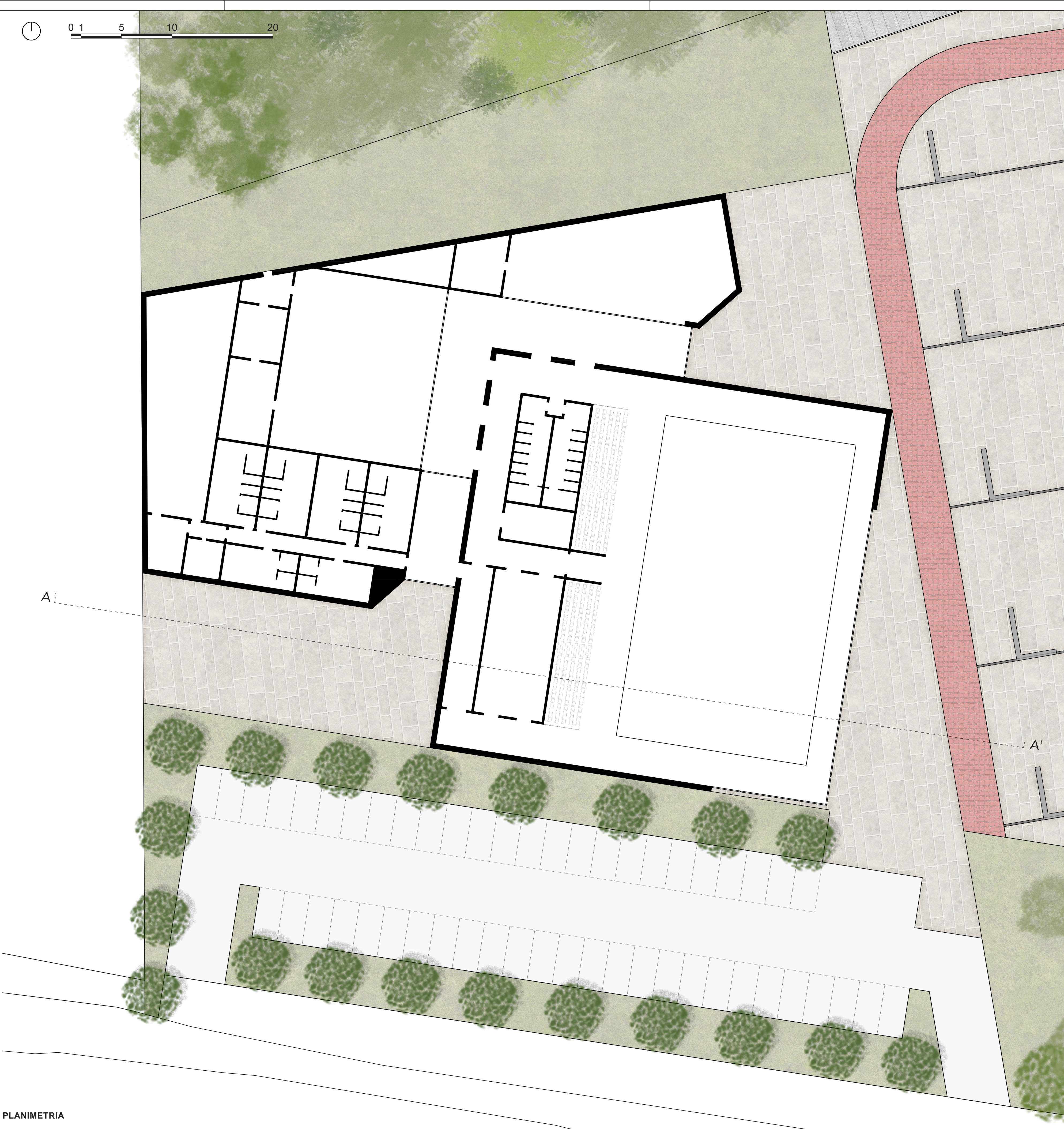
PLANIMETRIA
