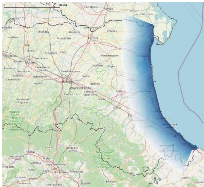
Figura 18 - gradiente di punteggio da associare alle tipologie di uso del suolo per tener conto dell'effetto brezza nel modello del SE microclima (+0,5 blu scuro fino a 0 bianco).
